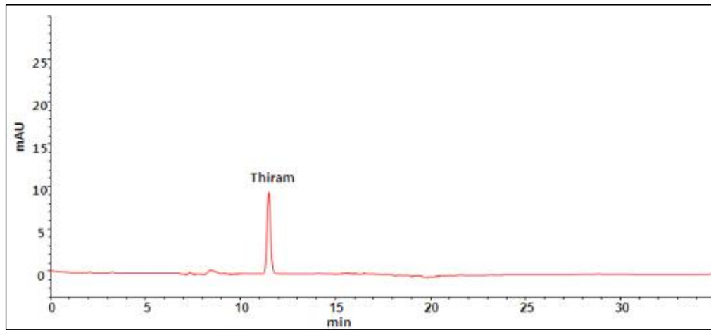
그림 2. 표준물질의 액체크로마토그램(Thiram)
